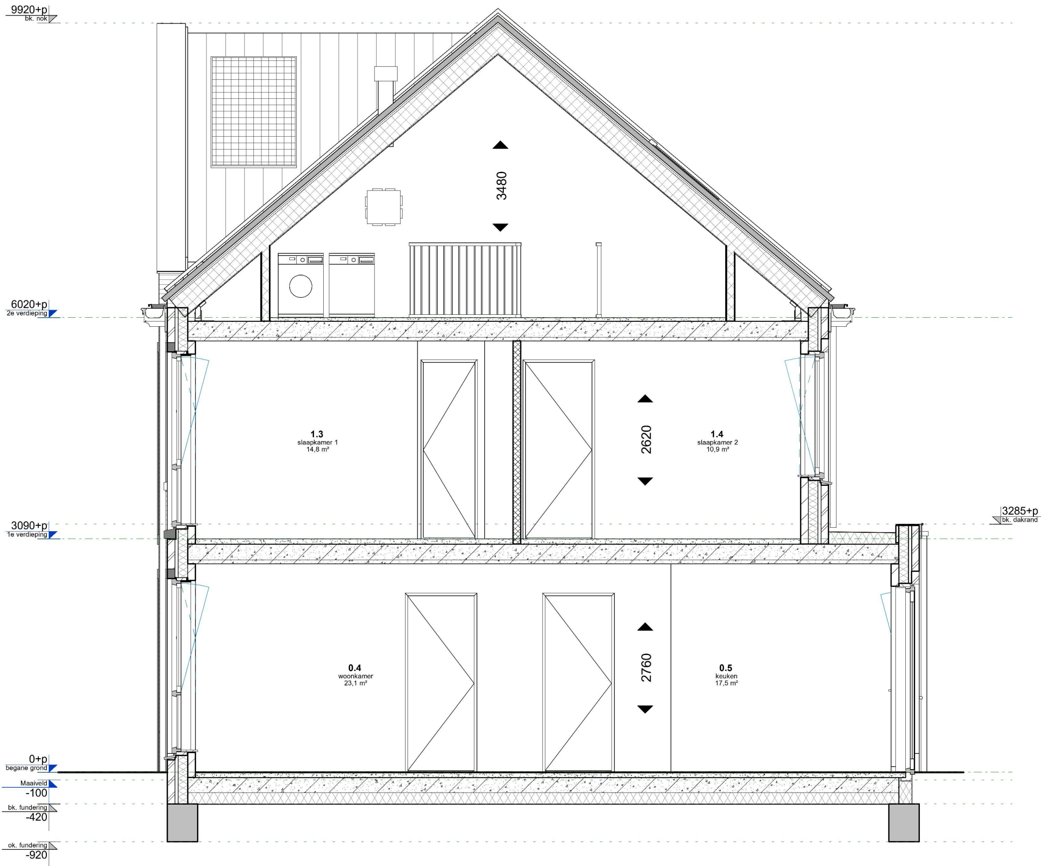
SCHAAL 1 DOORSNEDE
