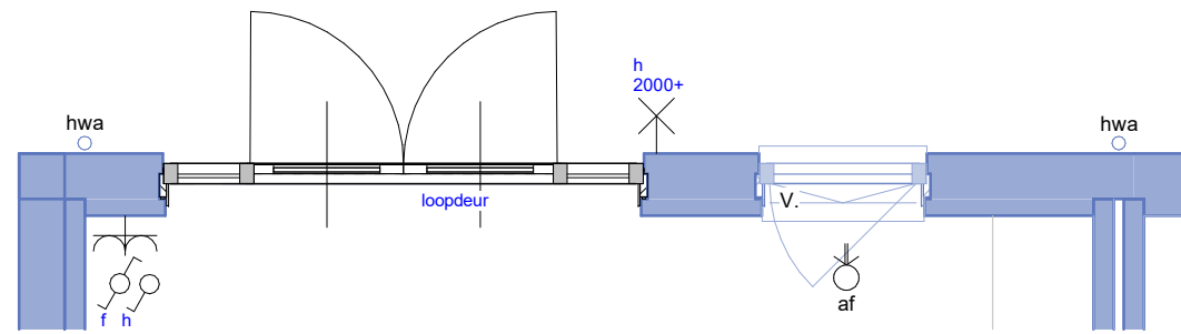
4 BEGANE GROND
