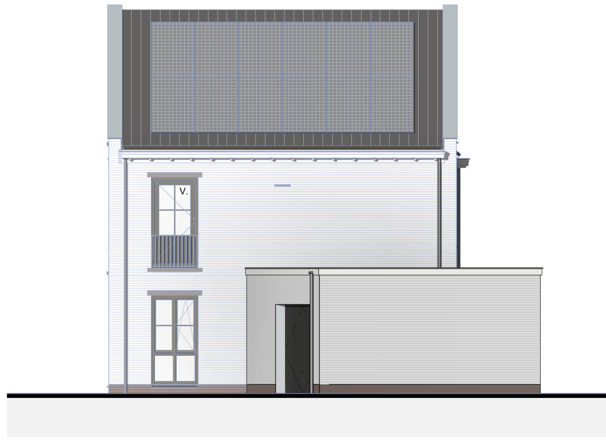
7 RECHTER GEVEL
