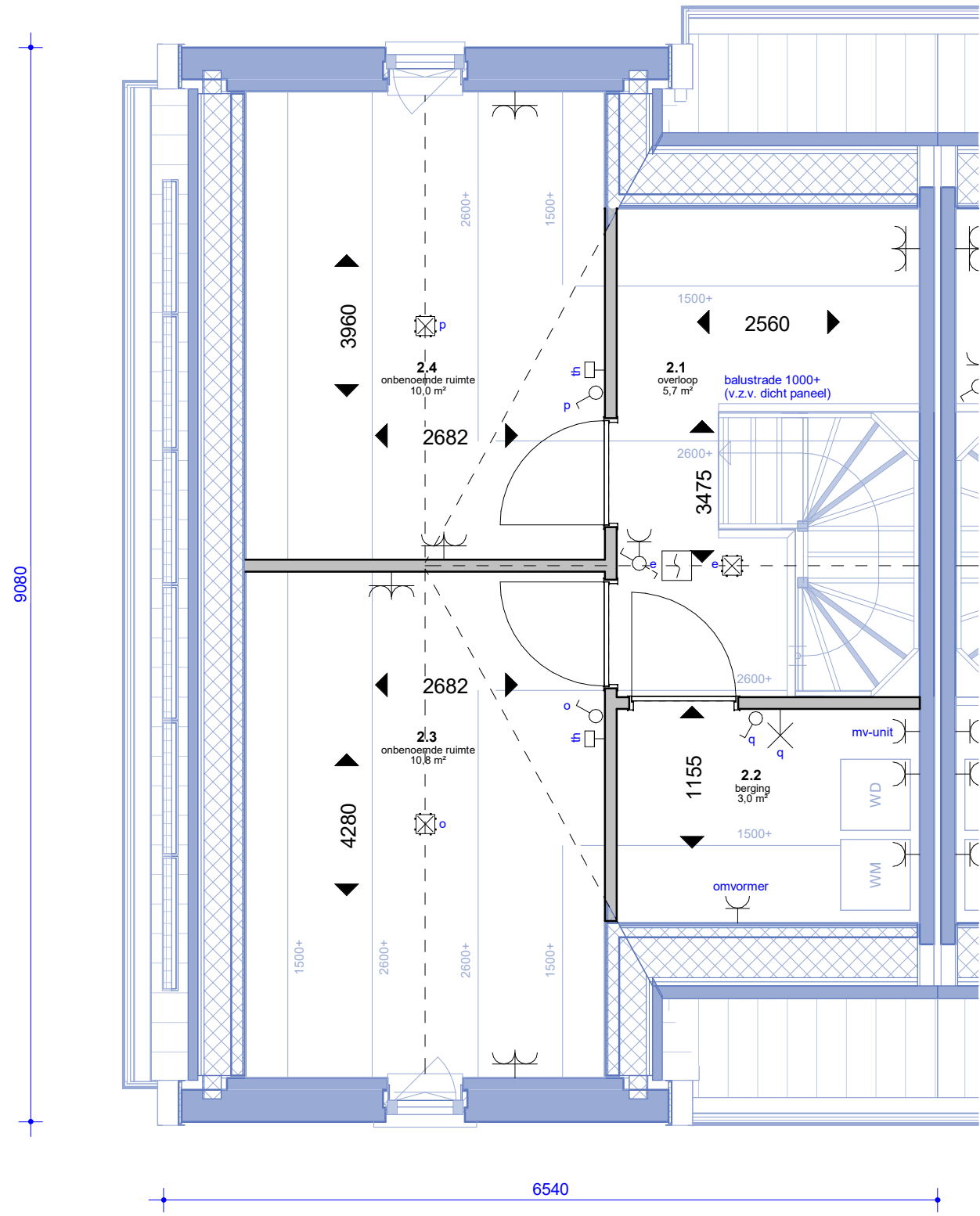
6 2e VERDIEPING
