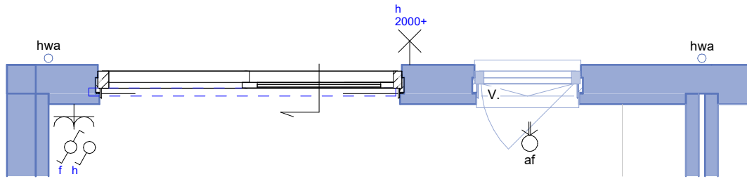
5 BEGANE GROND
