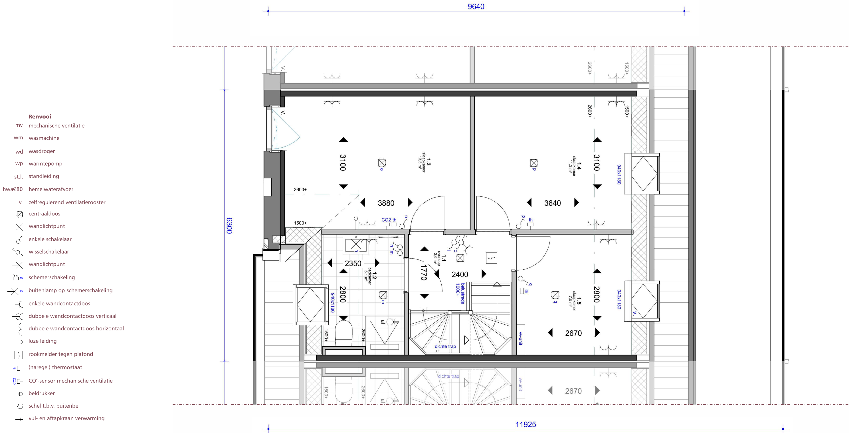
SCHAAL 1 OP 50 PLATTEGROND ~ EERSTE \
